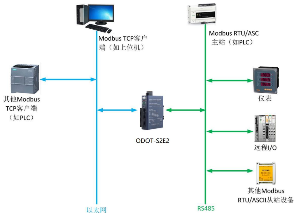
应用拓扑图
