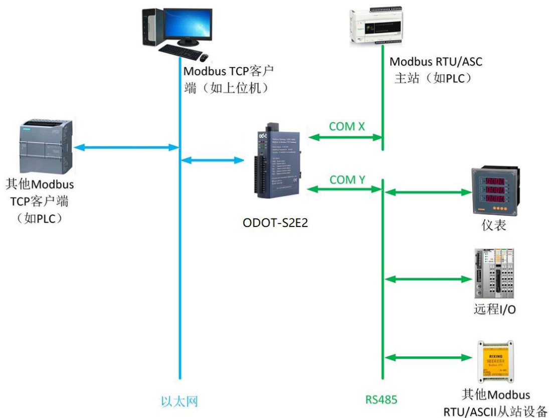
应用拓扑图
