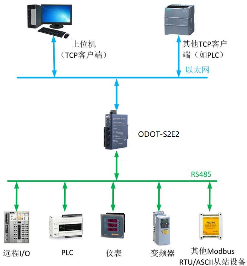
应用拓扑图
