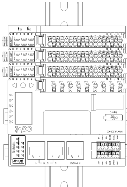
④垂直安装
