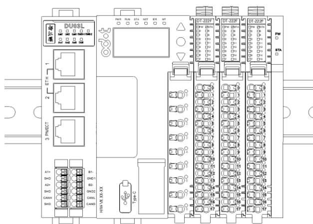
②水平安装
